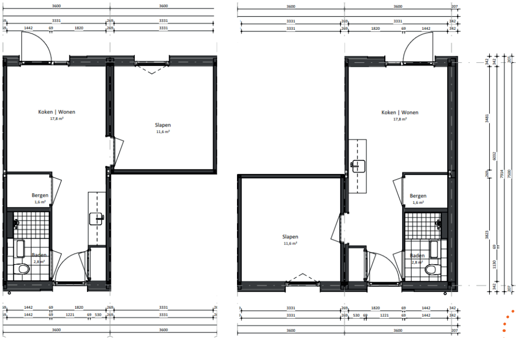
Plattegrond van type A en B
